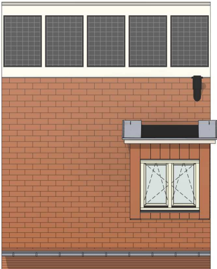
Voorgevel schaal 1:100
