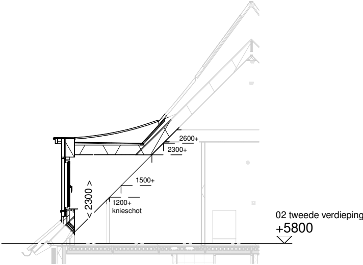
Doorsnede schaal 1:100
