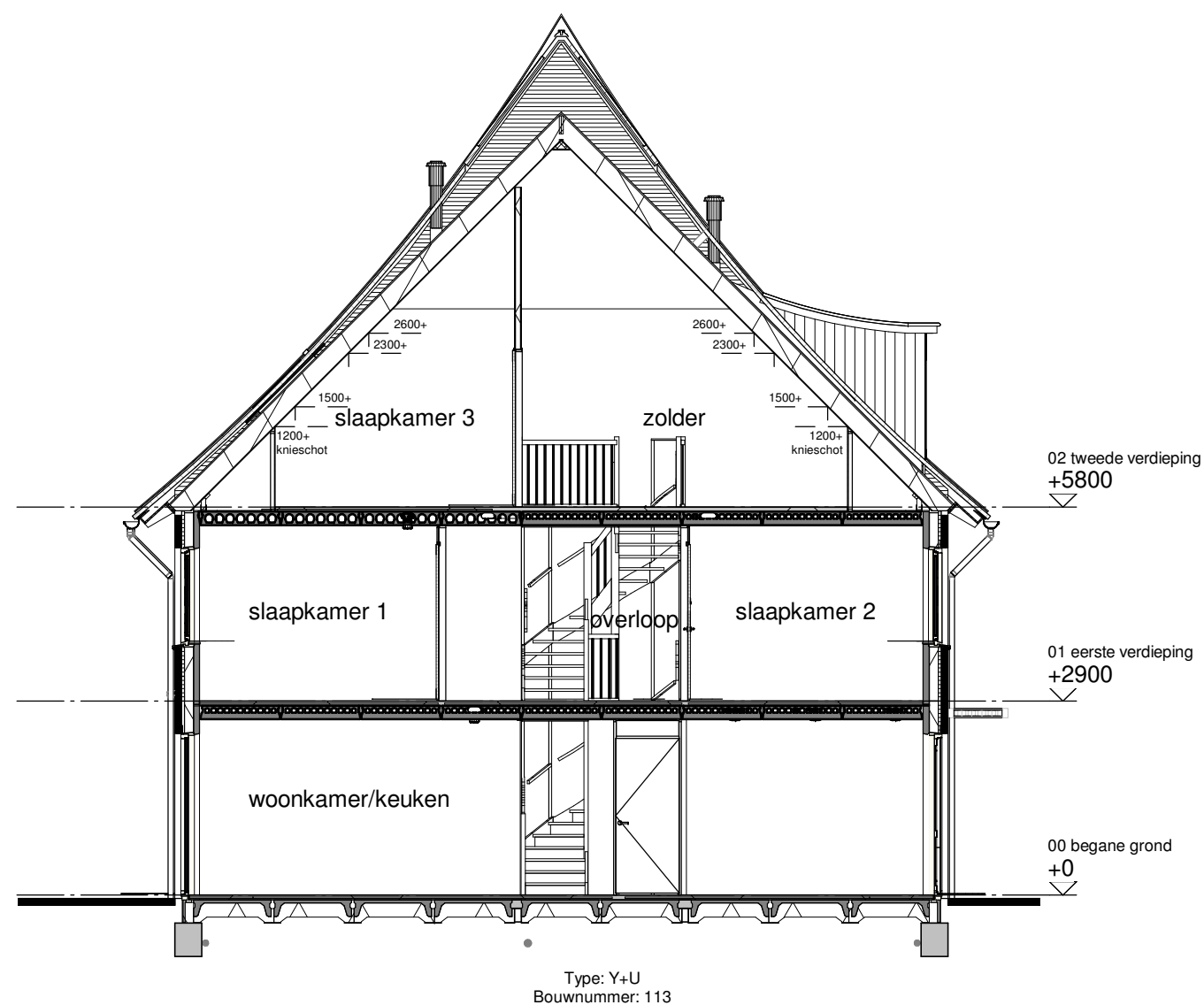
Doorsnede A
