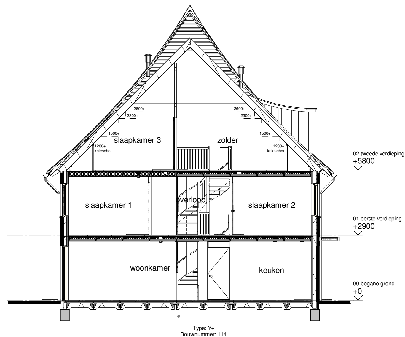
Doorsnede B
