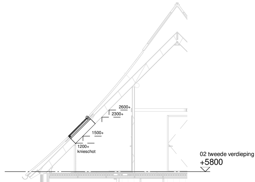
Doorsnede schaal 1:100
