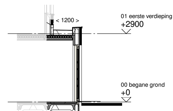
Doorsnede schaal 1:100
