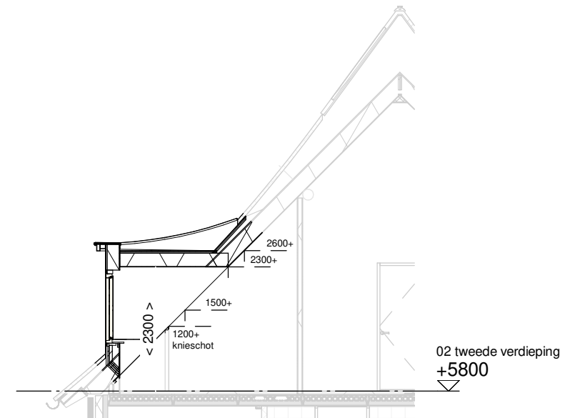
Doorsnede schaal 1:100
