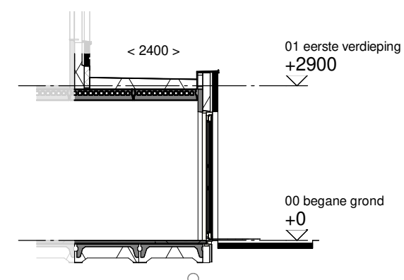
Doorsnede schaal 1:100
