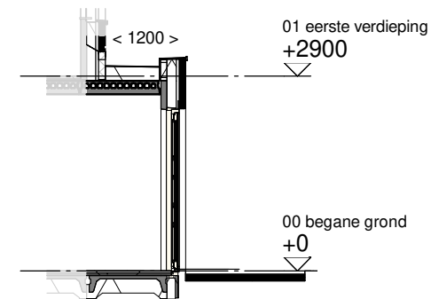
Doorsnede schaal 1:100
