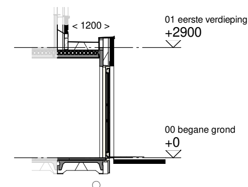
Doorsnede schaal 1:100
