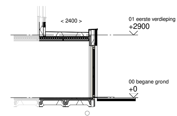
Doorsnede schaal 1:100
