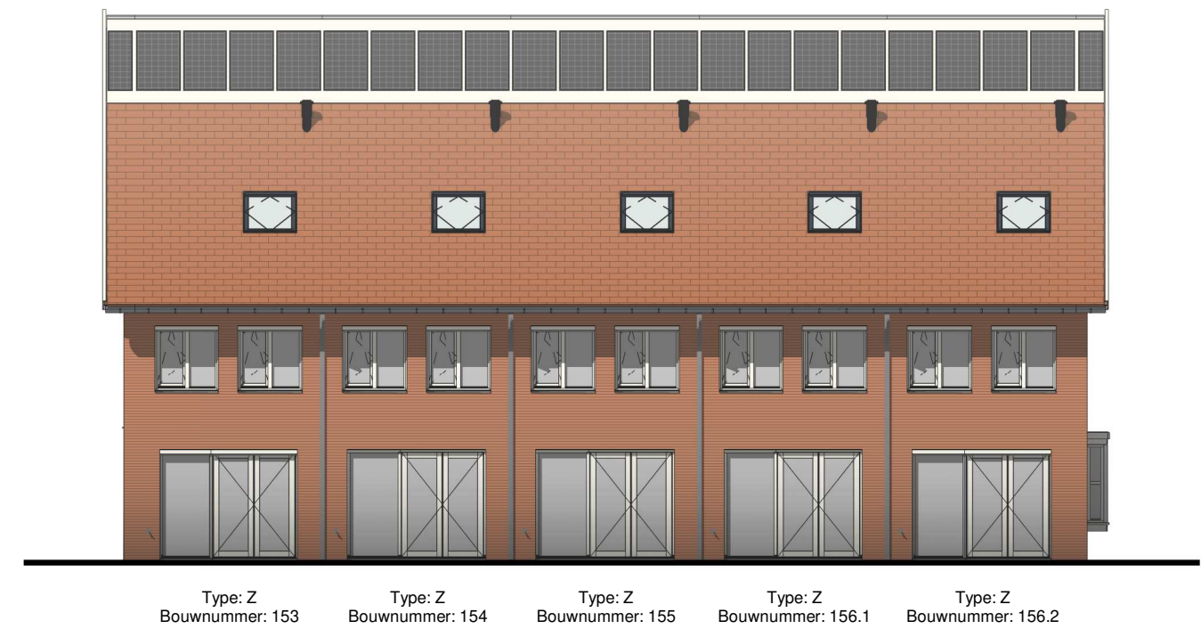
Achtergevel
