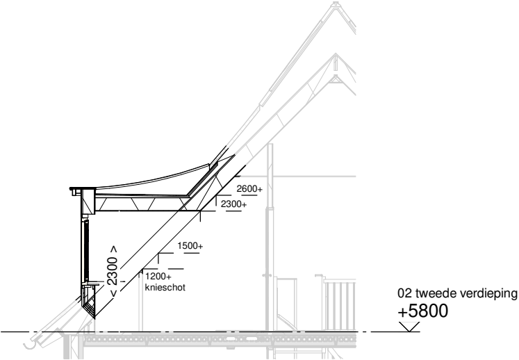
Doorsnede schaal 1:100
