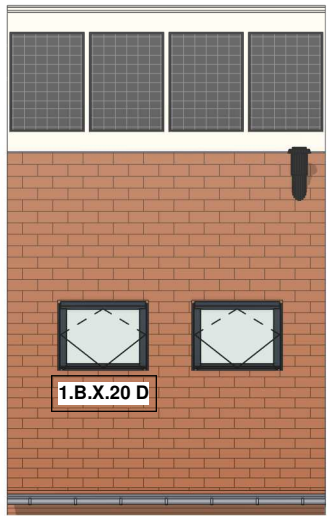
Voorgevel schaal 1:100
