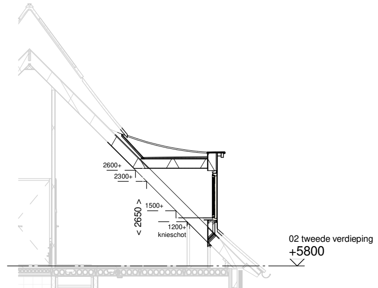
Doorsnede schaal 1:100
