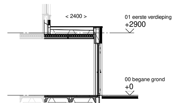
Doorsnede schaal 1:100
