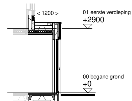
Doorsnede schaal 1:100
