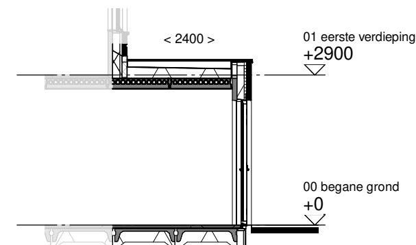
Doorsnede schaal 1:100
