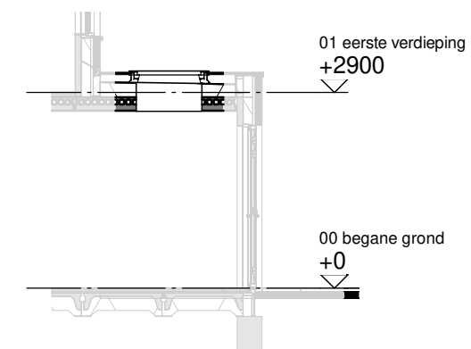
Doorsnede schaal 1:100
