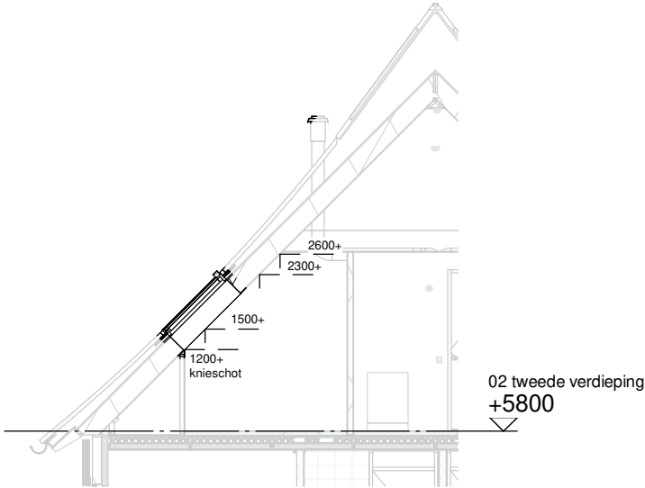
Doorsnede schaal 1:100
