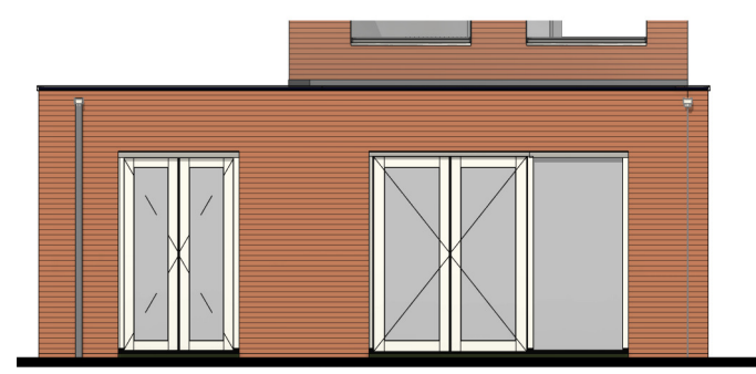
Achtergevel schaal 1:100
