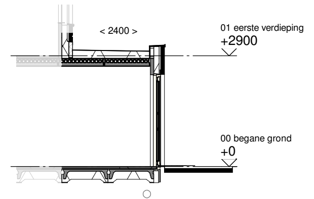
Doorsnede schaal 1:100
