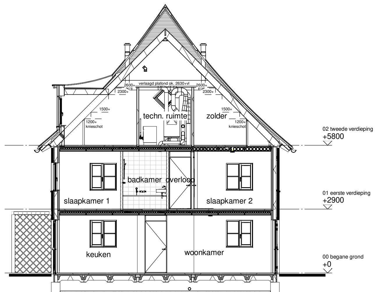
Doorsnede A
