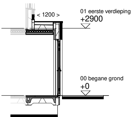
Doorsnede schaal 1:100
