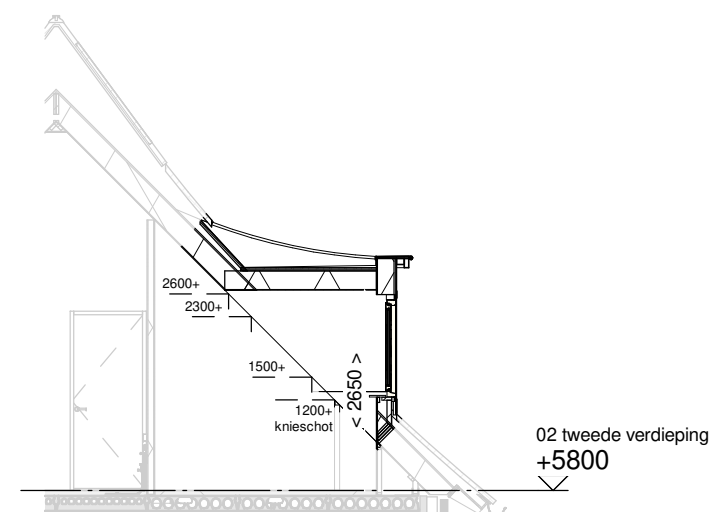
Achtergevel schaal 1:100
