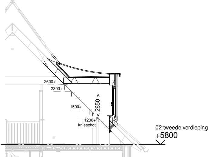
Doorsnede schaal 1:100
