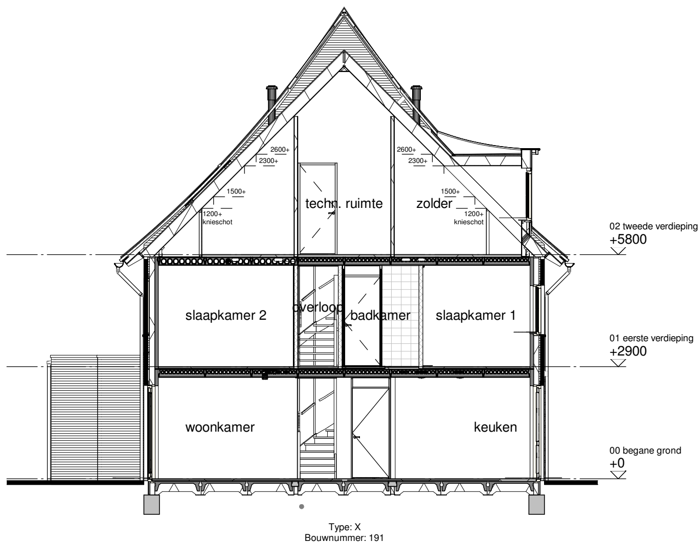
Doorsnede A
