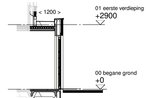
Doorsnede schaal 1:100
