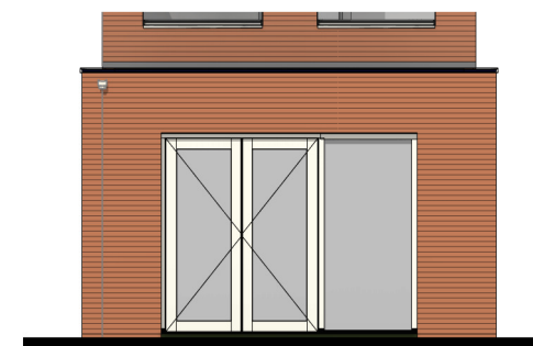
Achtergevel schaal 1:100
