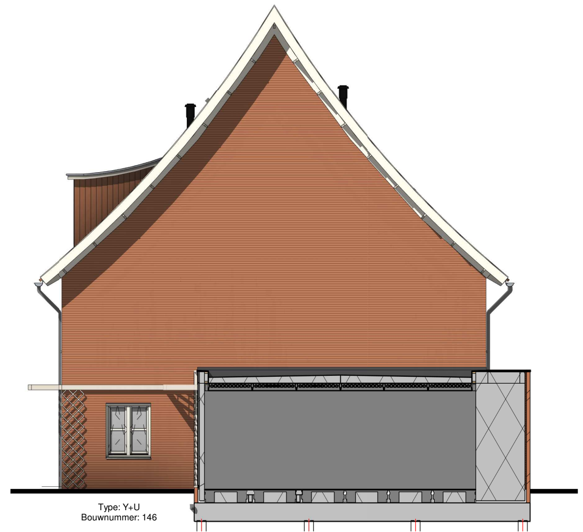
Rechter zijgevel
