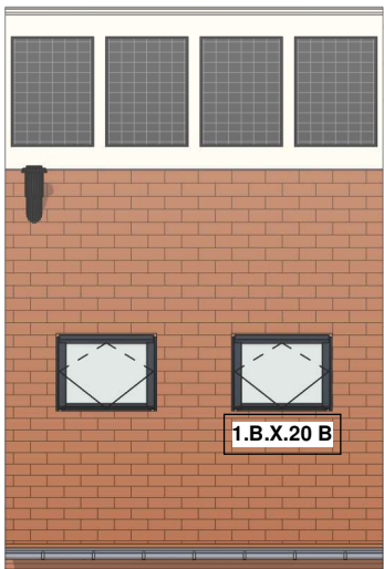
Achtergevel schaal 1:100
