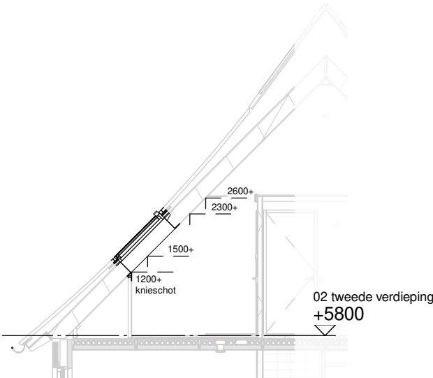
Doorsnede schaal 1:100
