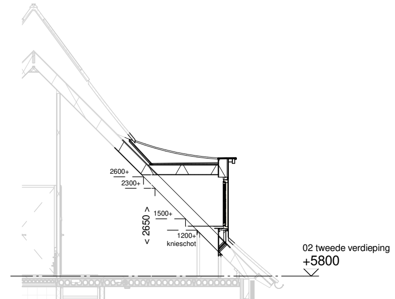
Doorsnede schaal 1:100
