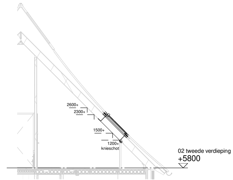
Doorsnede schaal 1:100
