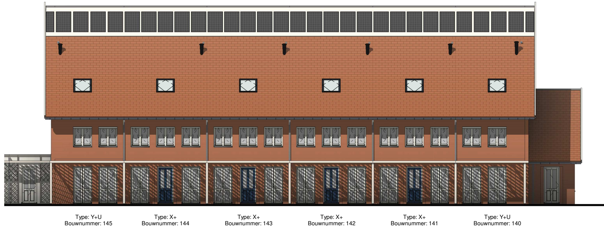
Voorgevel
