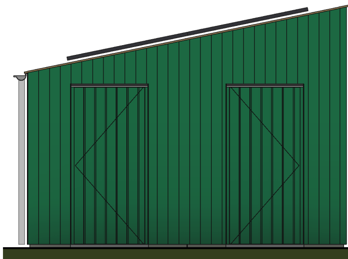
Linker zijgevel
