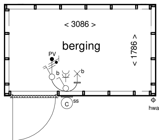
Begane grond
