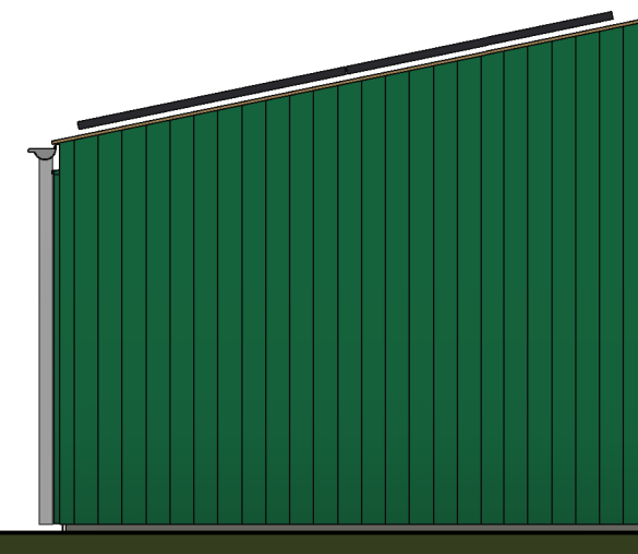
Rechter zijgevel
