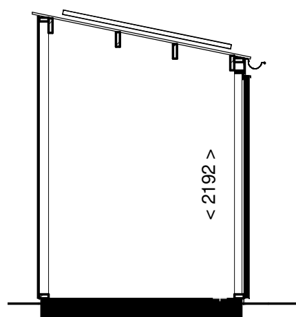
Doorsnede B-B
