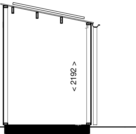
Doorsnede B-B
