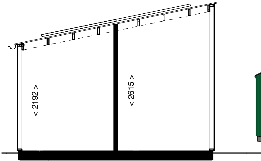
Doorsnede B-B
