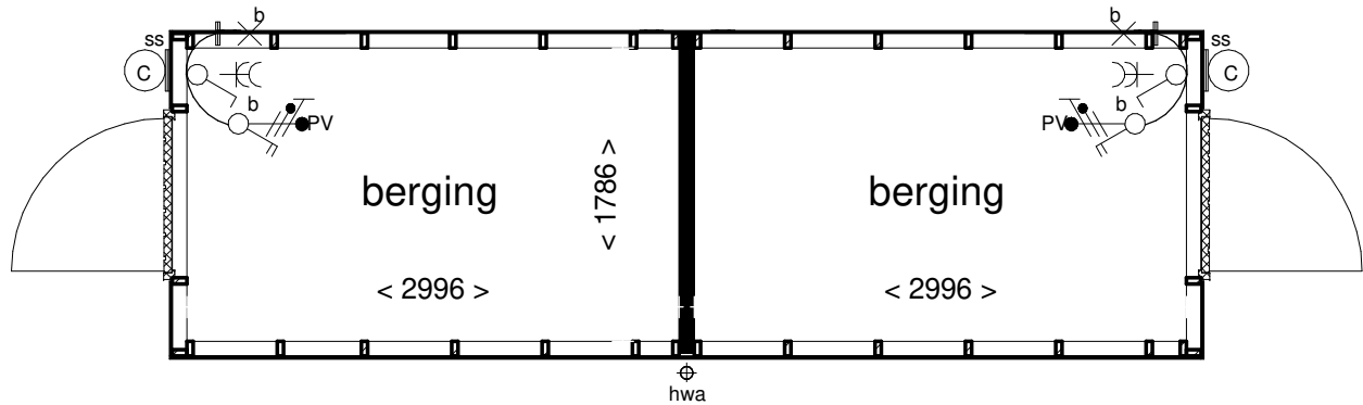
Begane grond
