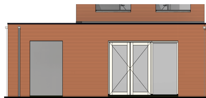
Achtergevel schaal 1:100
