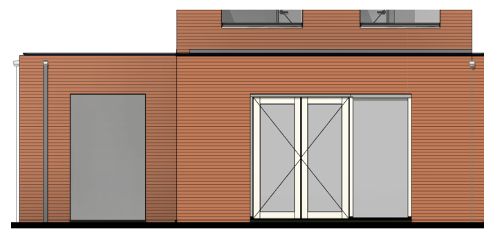
Achtergevel schaal 1:100
