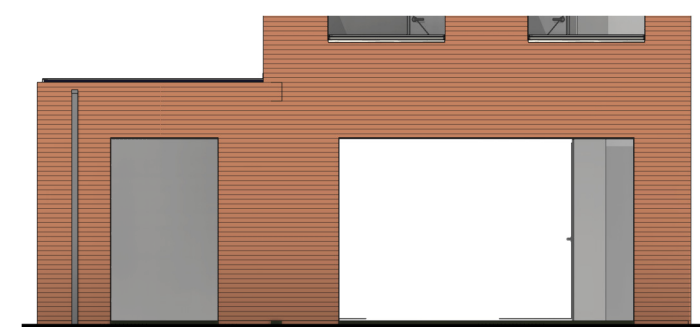
Achtergevel schaal 1:100
