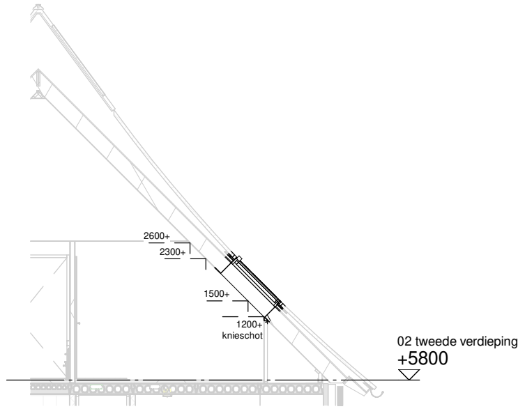
Doorsnede schaal 1:100
