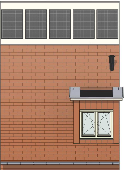
Voorgevel schaal 1:100
