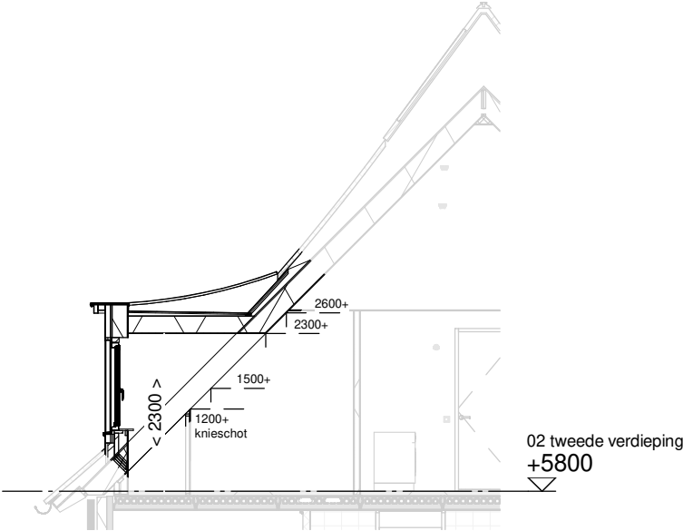
Doorsnede schaal 1:100
