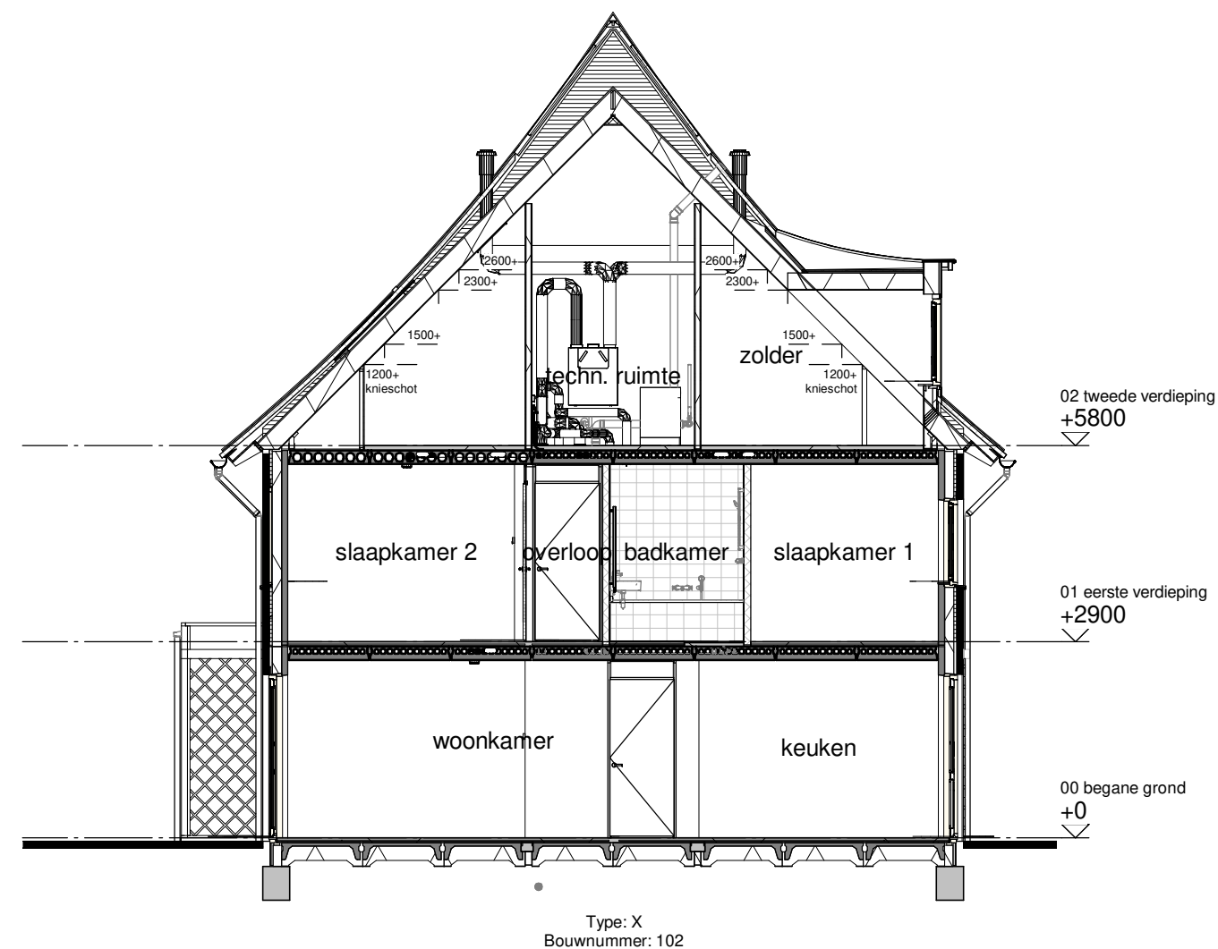
Doorsnede B
