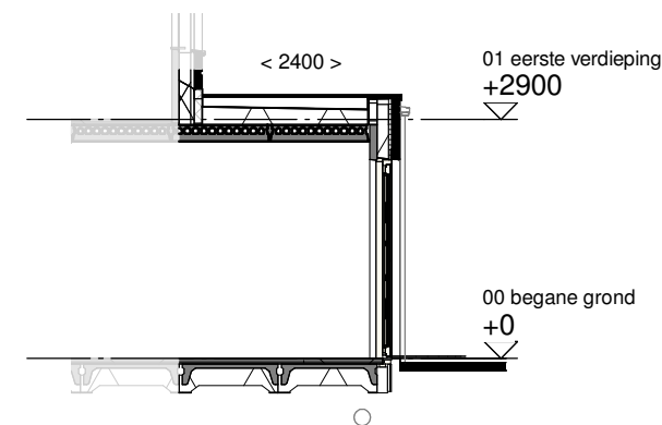
Doorsnede schaal 1:100
