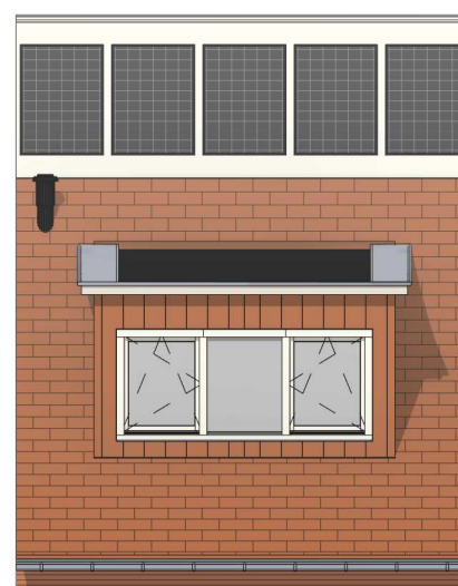
Achtergevel schaal 1:100
