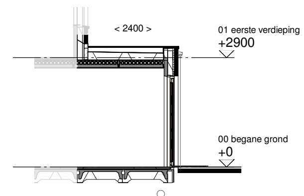
Doorsnede schaal 1:100
