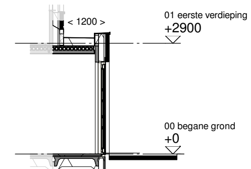
Doorsnede schaal 1:100
