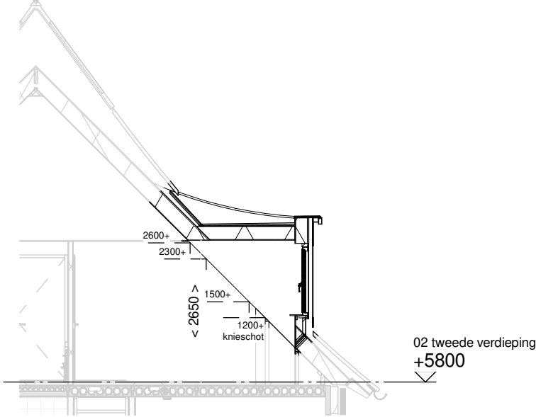
Doorsnede schaal 1:100
