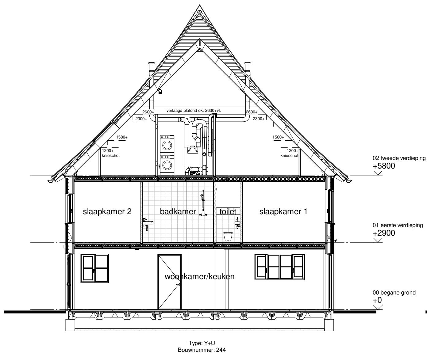
Doorsnede A
