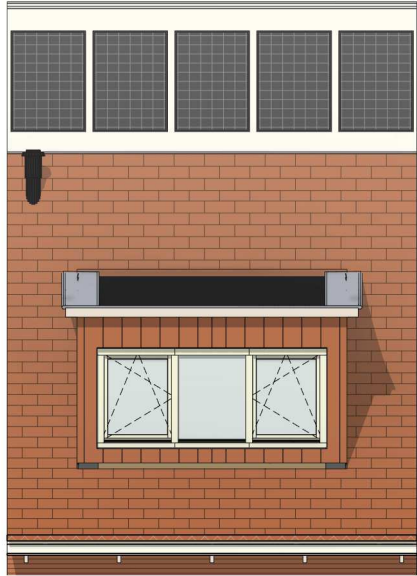
Achtergevel schaal 1:100
