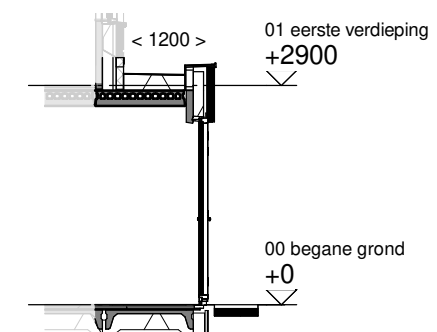
Doorsnede schaal 1:100
