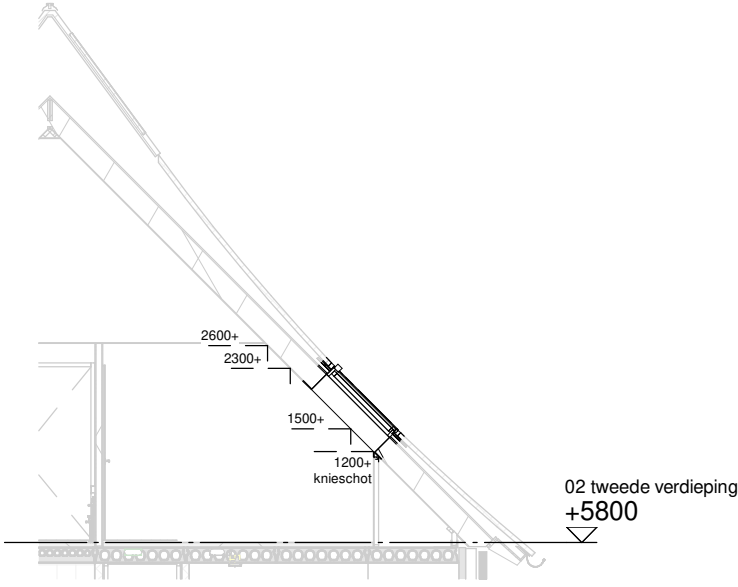
Doorsnede schaal 1:100
