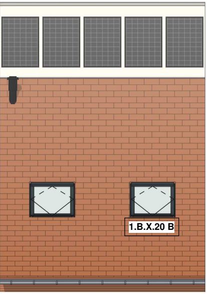
Achtergevel schaal 1:100
