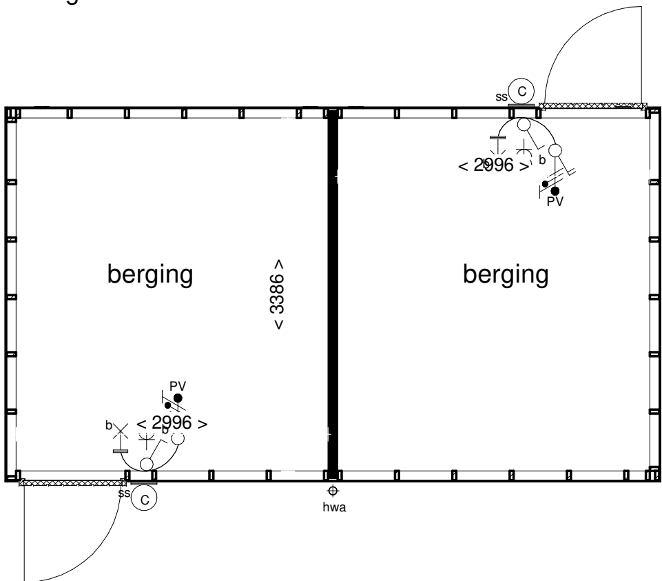
Begane grond
