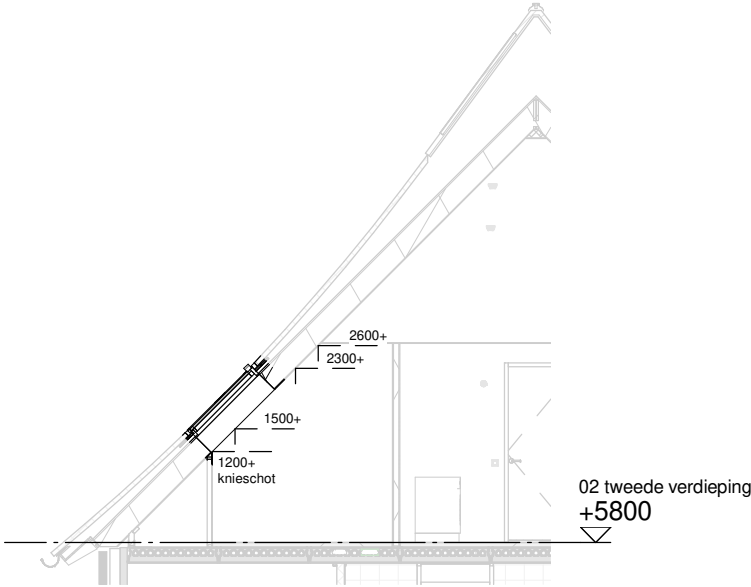
Doorsnede schaal 1:100
