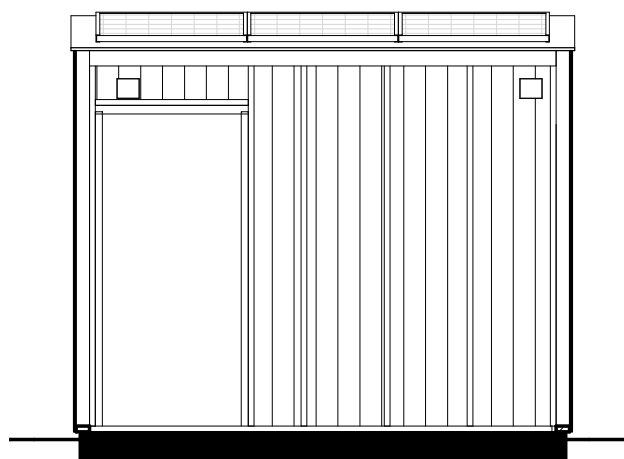
Doorsnede A-A
