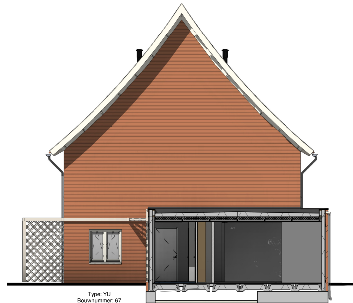
Rechter zijgevel
