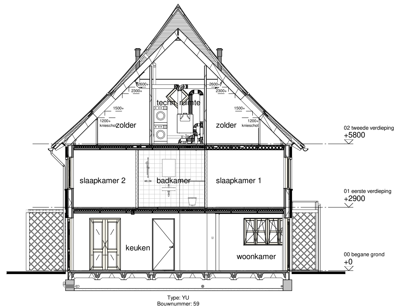
Doorsnede B
