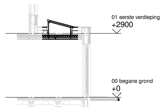
Doorsnede schaal 1:100
