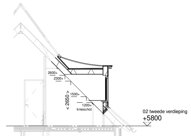
Doorsnede schaal 1:100
