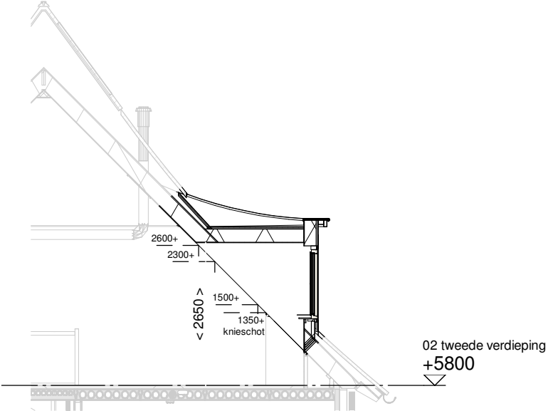
Doorsnede schaal 1:100
