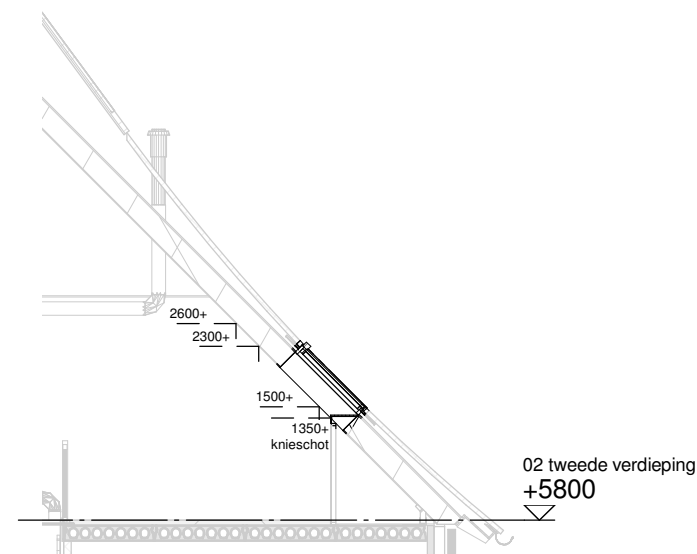
Doorsnede schaal 1:100
