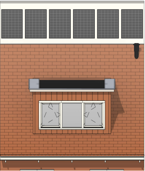
Achtergevel schaal 1:100
