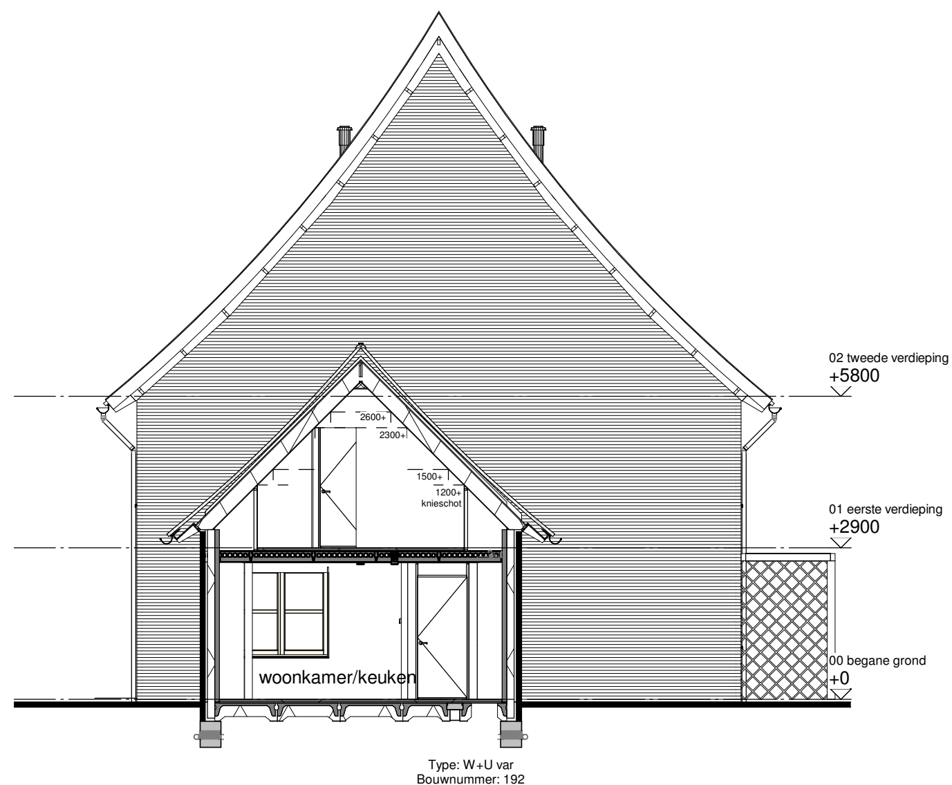
Doorsnede A
