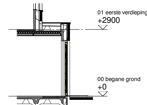
Doorsnede schaal 1:100
