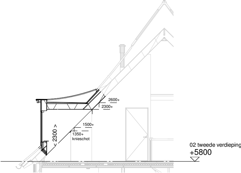
Doorsnede schaal 1:100
