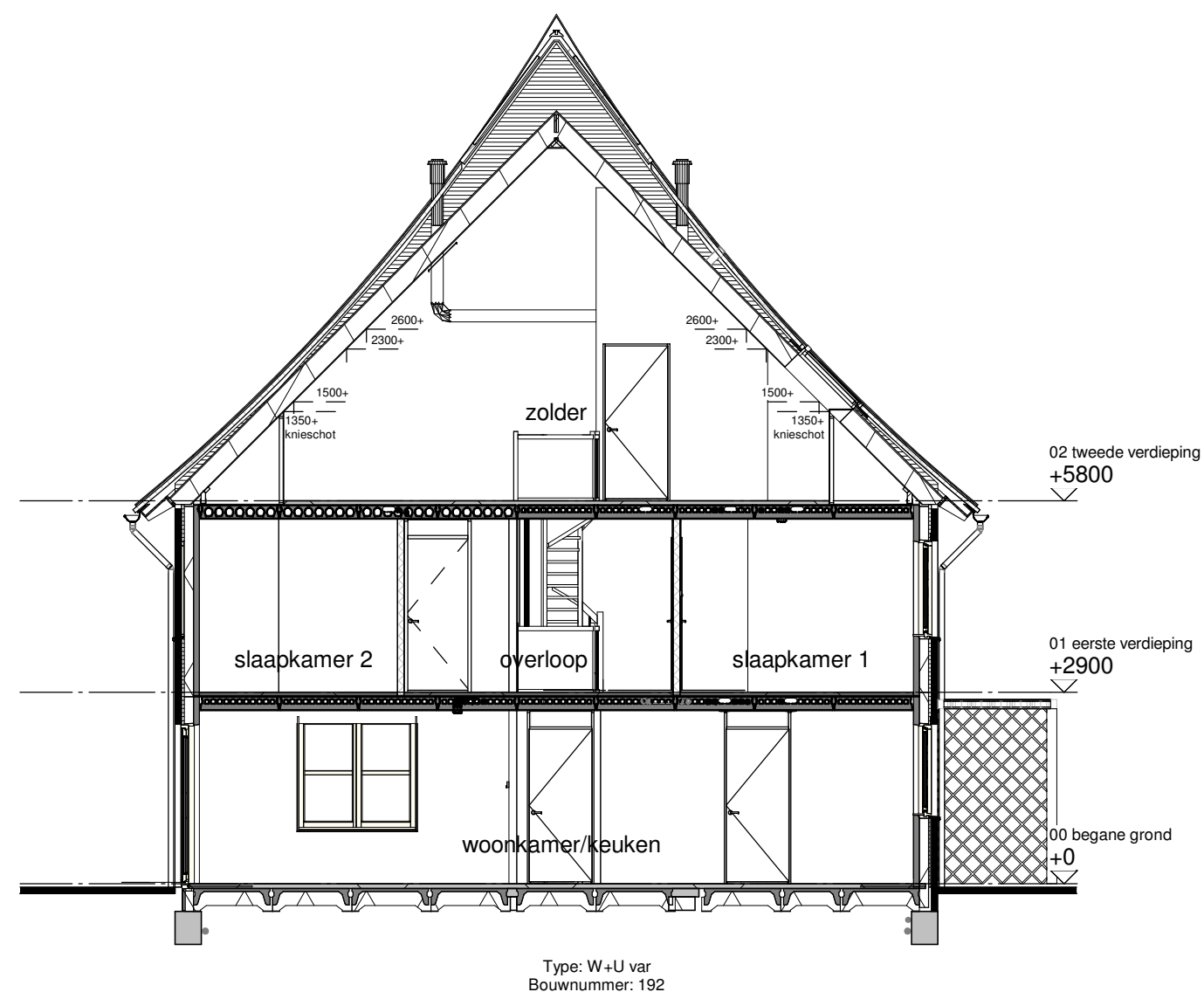
Doorsnede B
