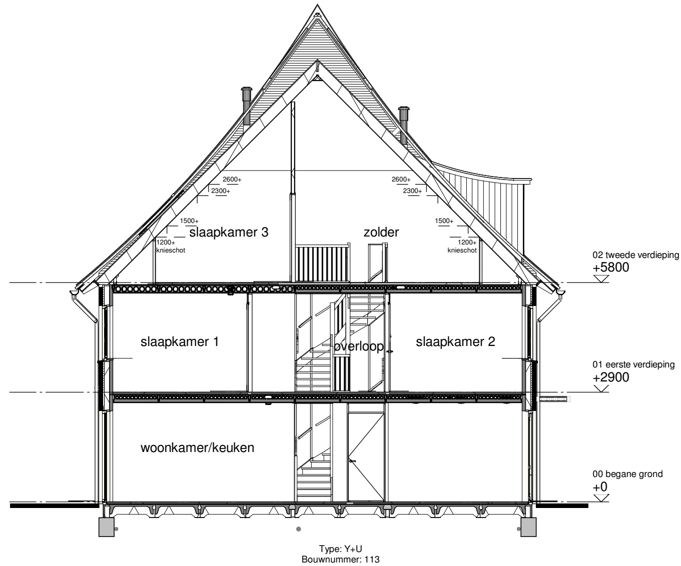
Doorsnede A
