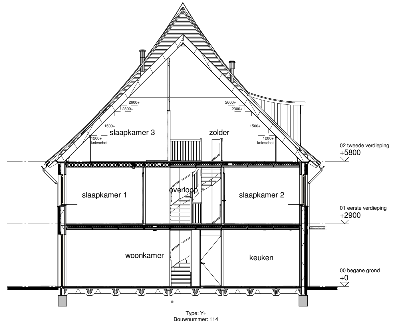
Doorsnede B
