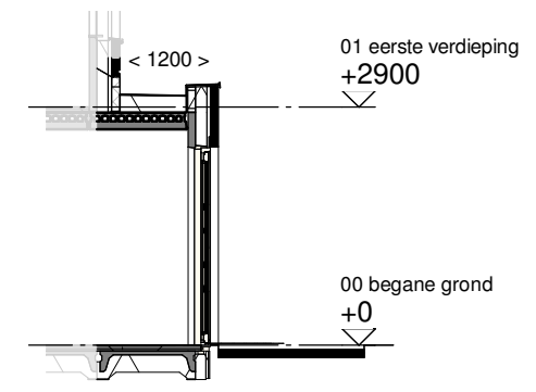
Doorsnede schaal 1:100
