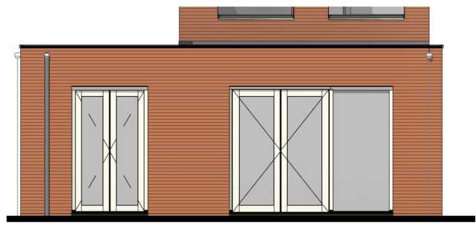
Achtergevel schaal 1:100
