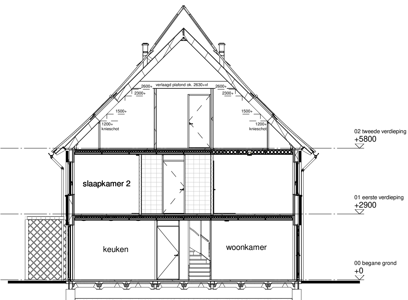
Doorsnede B Type: YU Bouwnummer: 209
