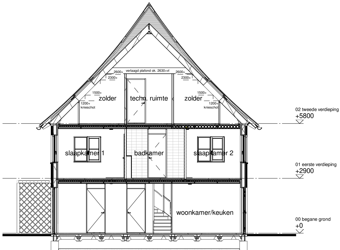
Doorsnede A Type: Z45 Bouwnummer: 218
