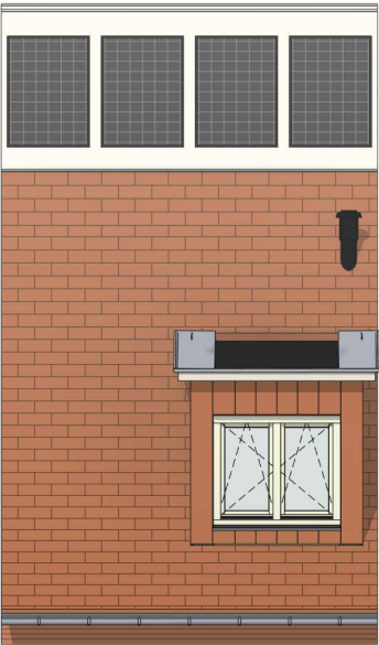
Voorgevel schaal 1:100
