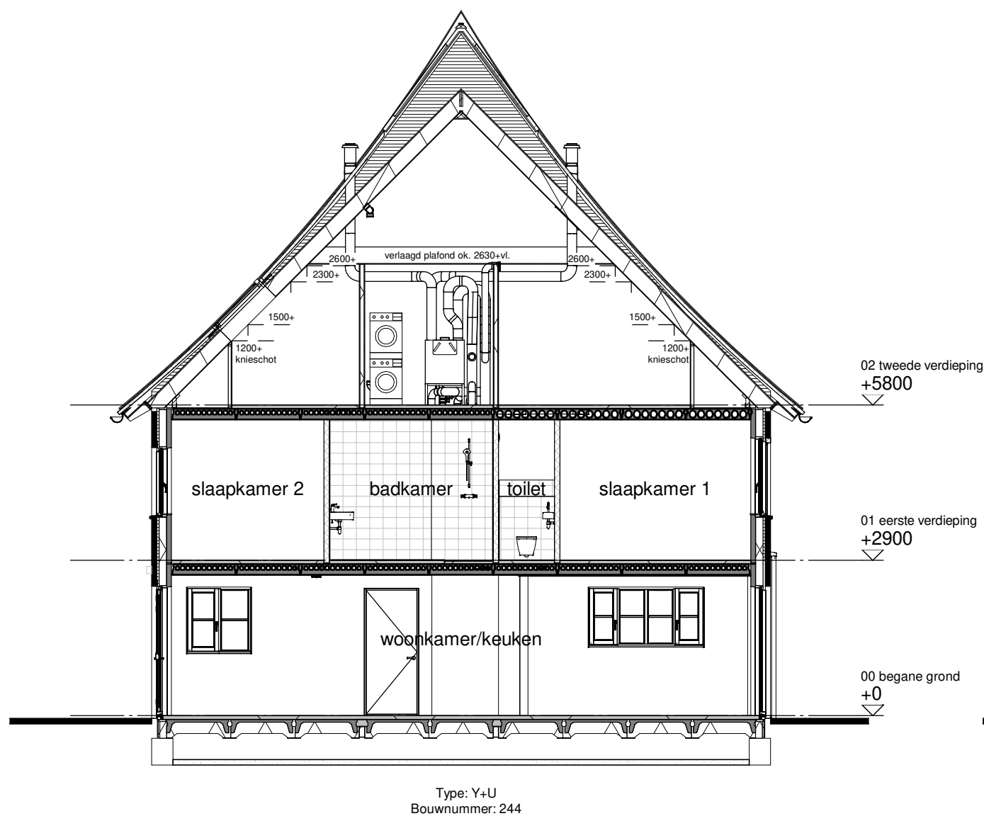
Doorsnede A
