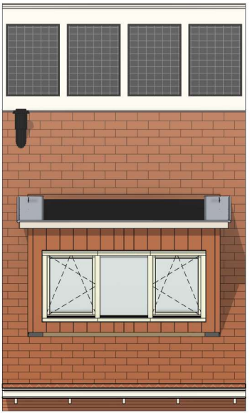
Achtergevel schaal 1:100
