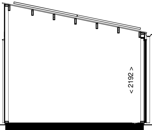
Doorsnede B-B
