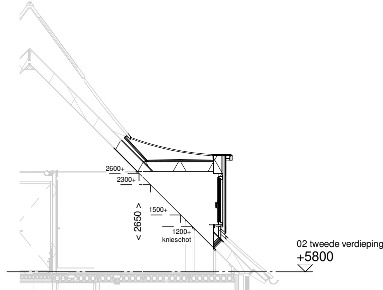
Doorsnede schaal 1:100
