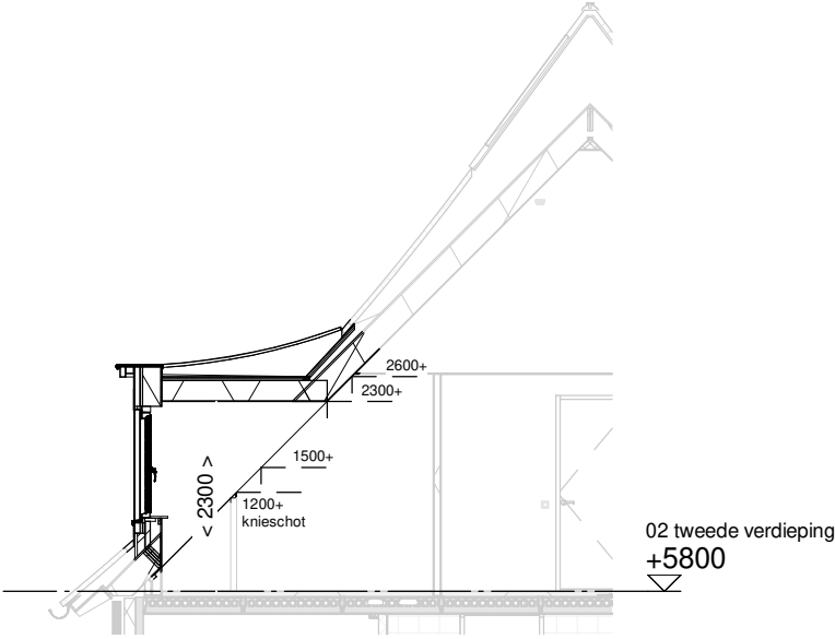
Doorsnede schaal 1:100
