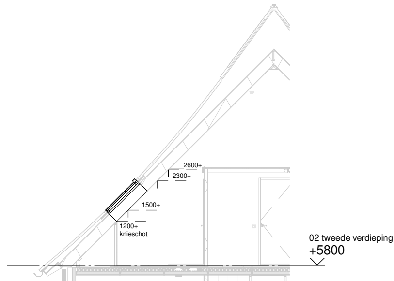
Doorsnede schaal 1:100
