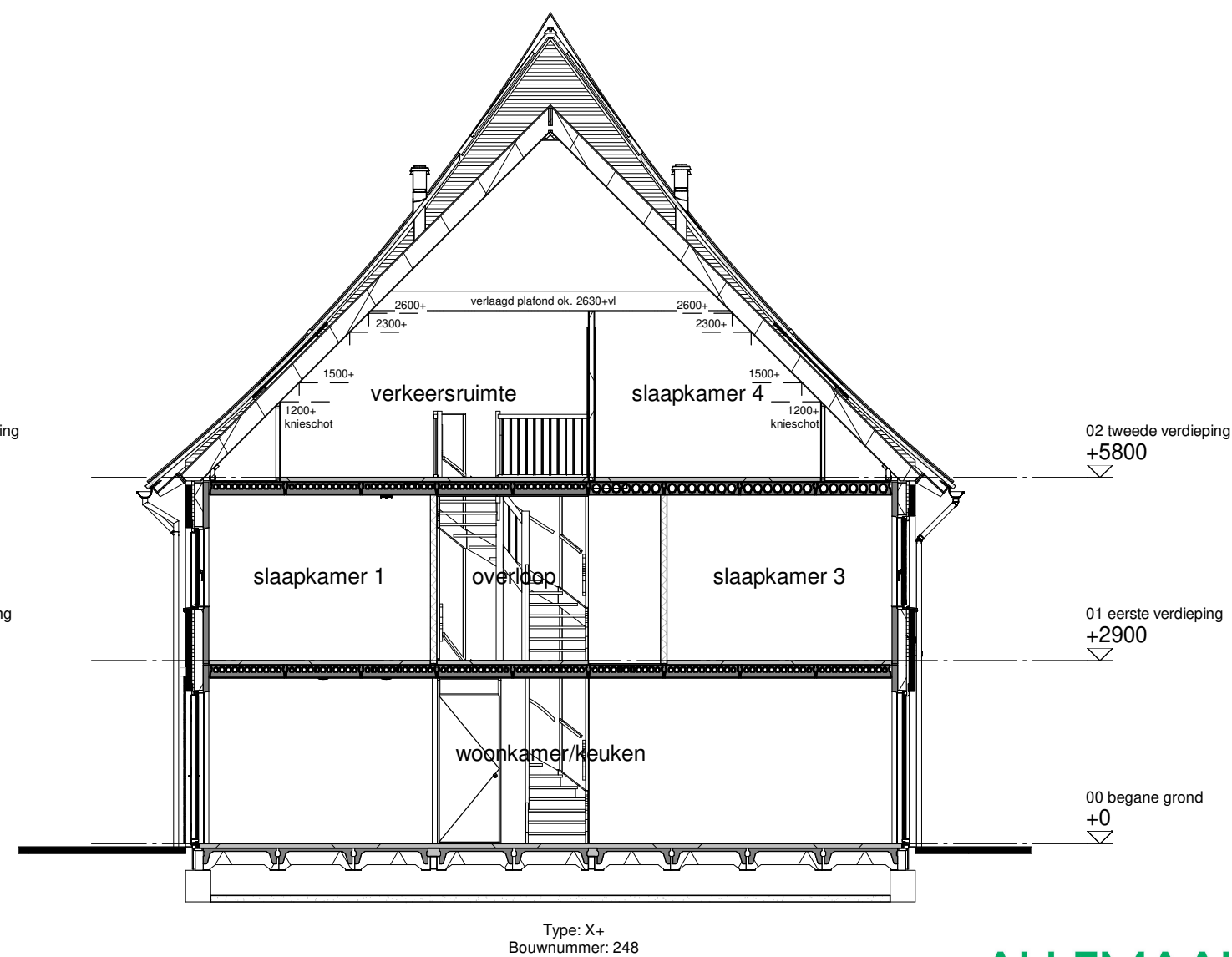
Doorsnede B
