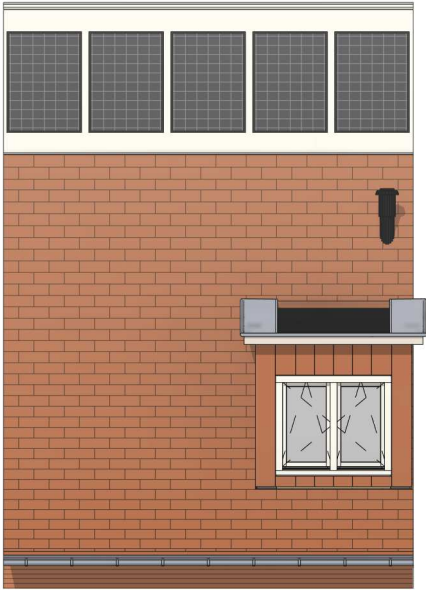
Achtergevel schaal 1:100
