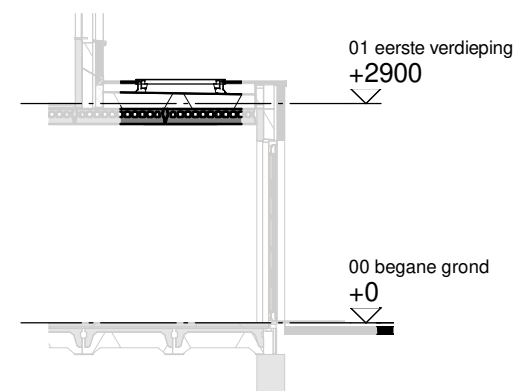
Doorsnede schaal 1:100
