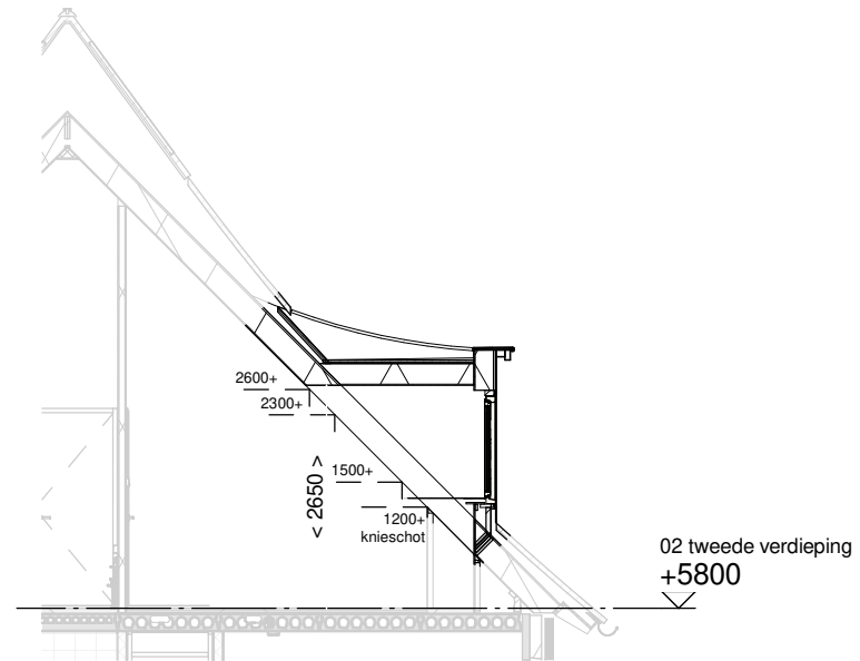
Doorsnede schaal 1:100
