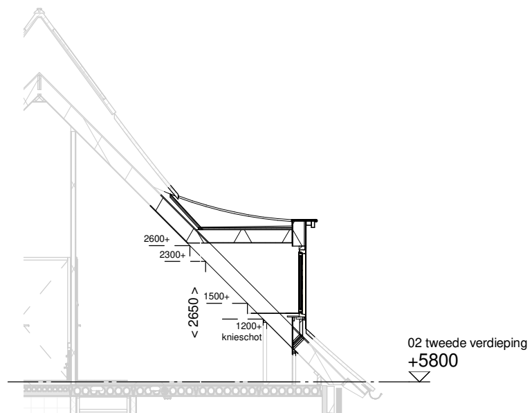
Doorsnede schaal 1:100
