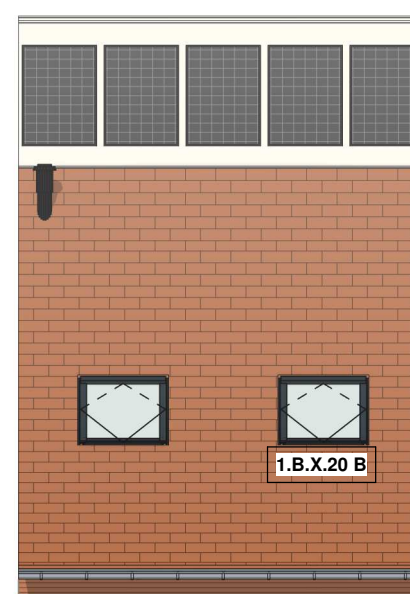
Achtergevel schaal 1:100
