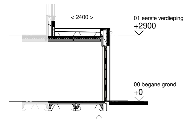
Doorsnede schaal 1:100
