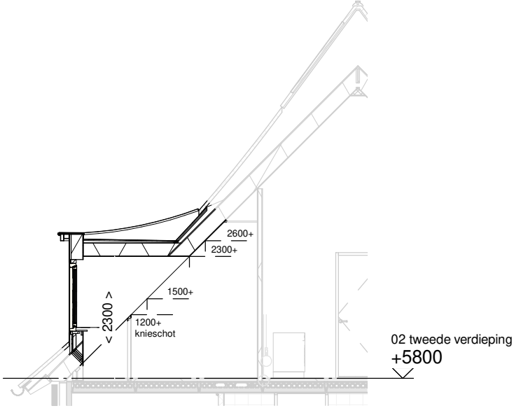
Doorsnede schaal 1:100
