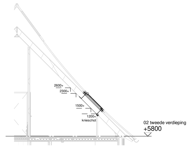
Doorsnede schaal 1:100
