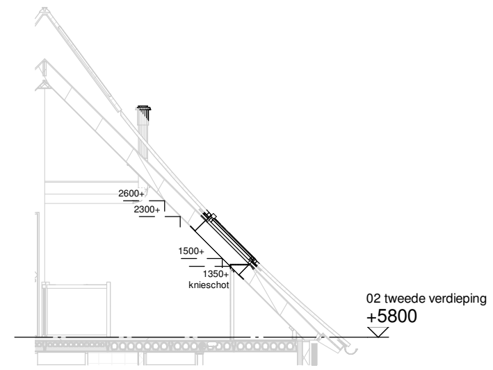
Doorsnede schaal 1:100
