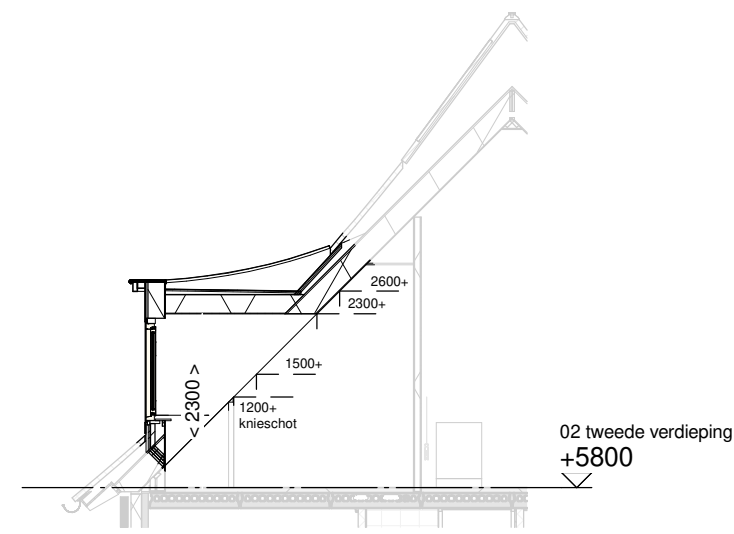
Doorsnede schaal 1:100
