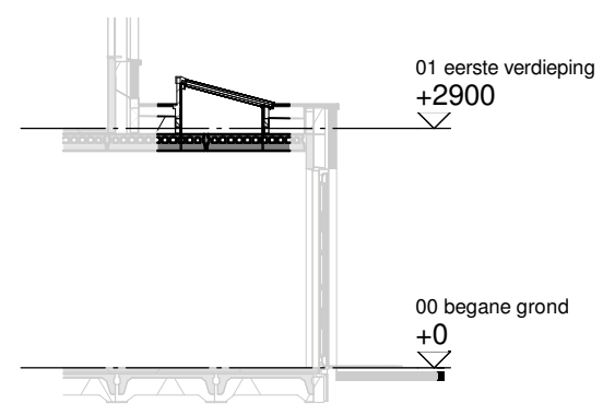
Doorsnede schaal 1:100
