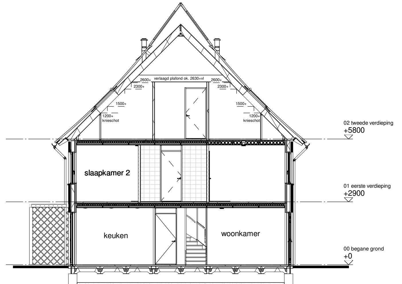
Doorsnede B
