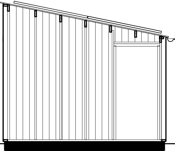
Doorsnede B-B
