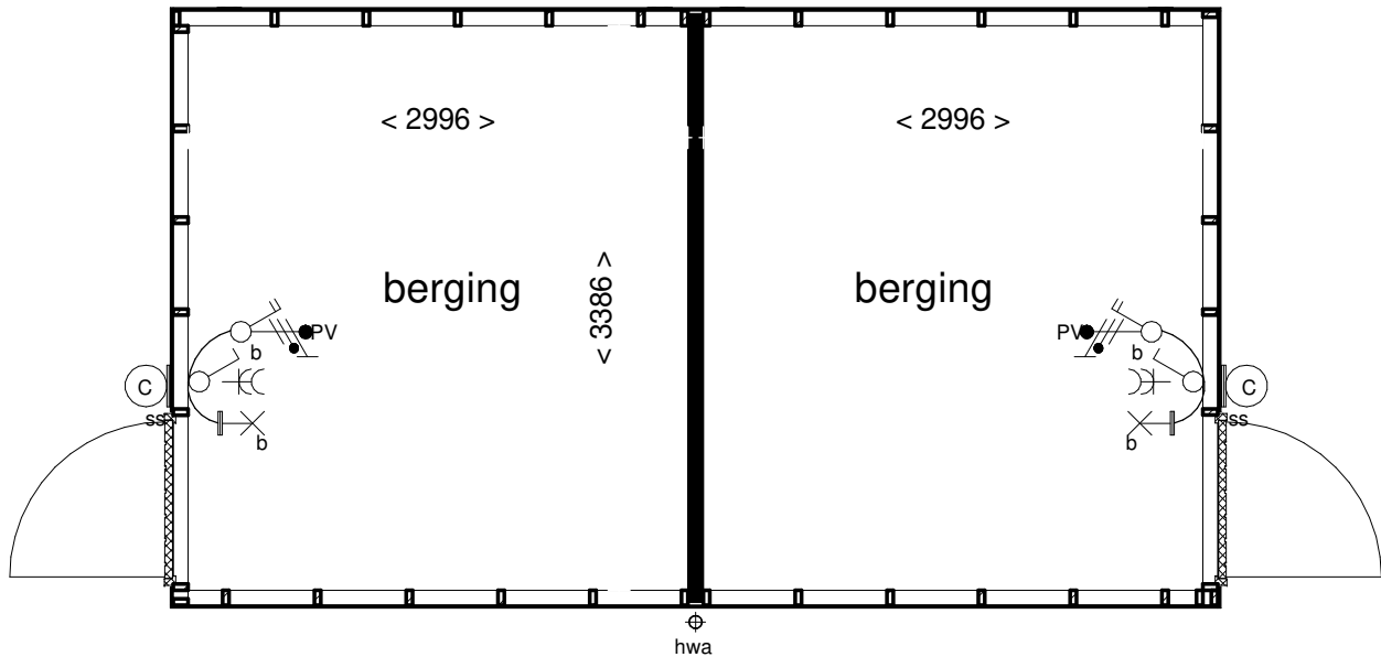
Begane grond
