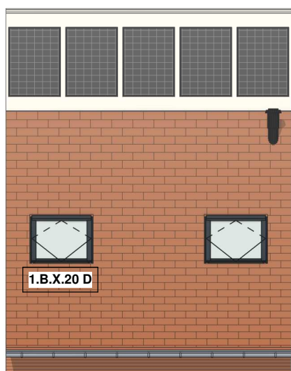
Voorgevel schaal 1:100
