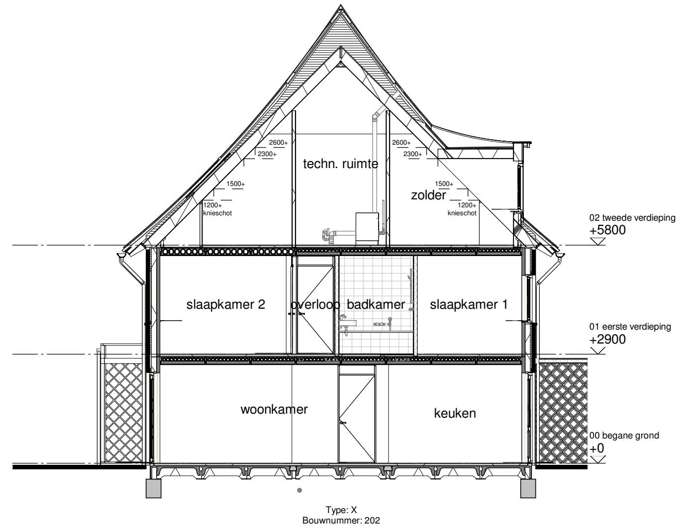
Doorsnede B
