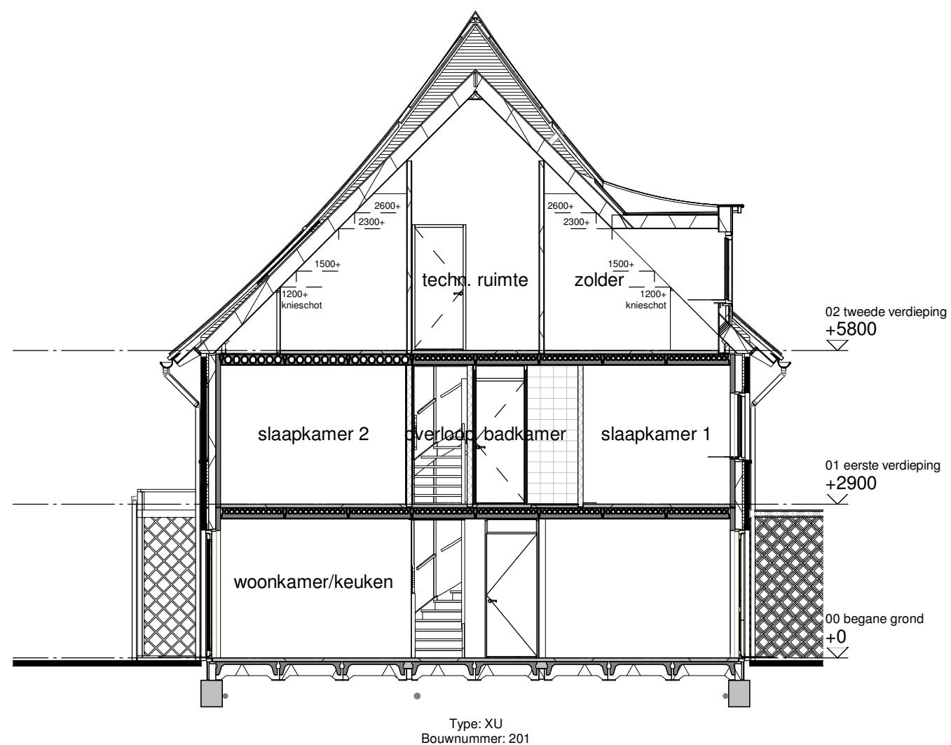
Doorsnede A
