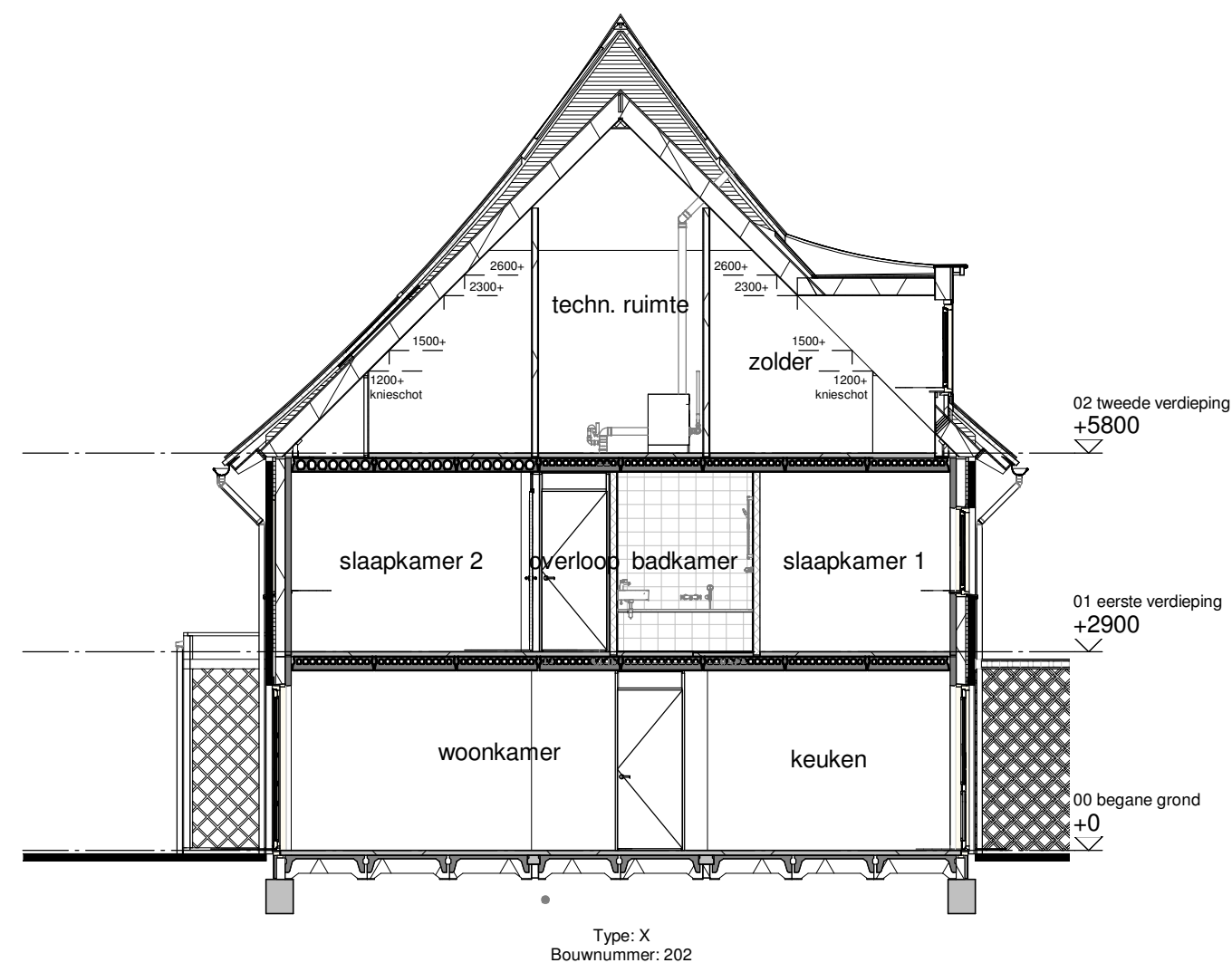
Doorsnede B
